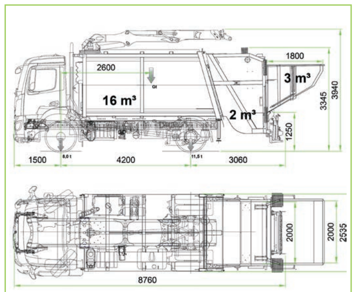
ECONIC - niskopodno vozilo s kranom u funkciji
