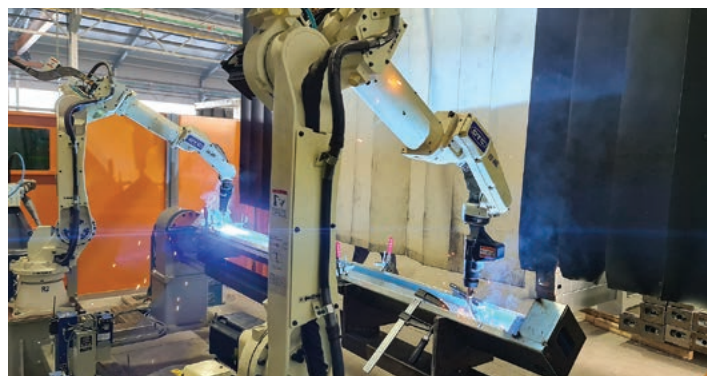
Robotsko lasersko zavarivanje
