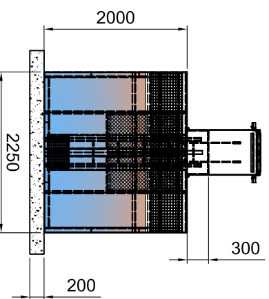
Regulacija kliznih grla vijcima M12x25
